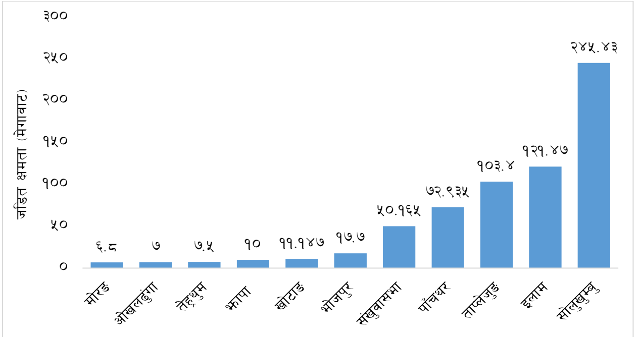
चार्ट ६.१ : जिल्लागत विद्युत उत्पादनको अवस्था (जडित क्षमता)
